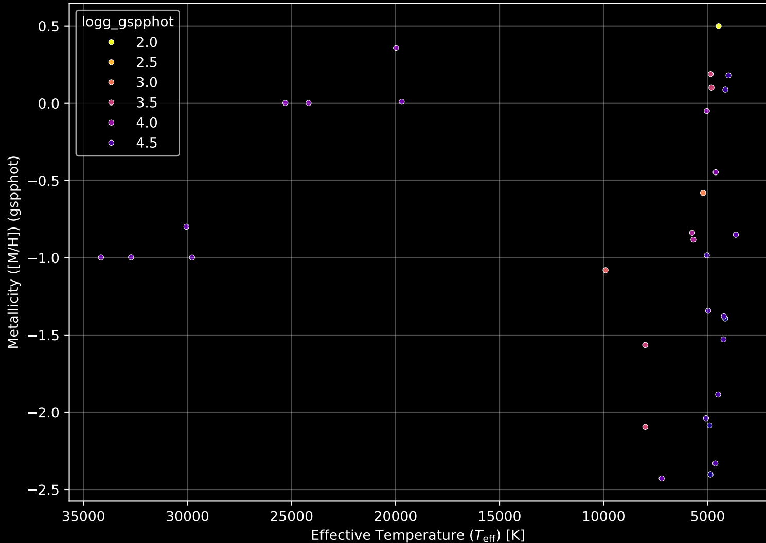
GALAH DR4 Field: [-7] Stellar Population Parameters (n= 33)
