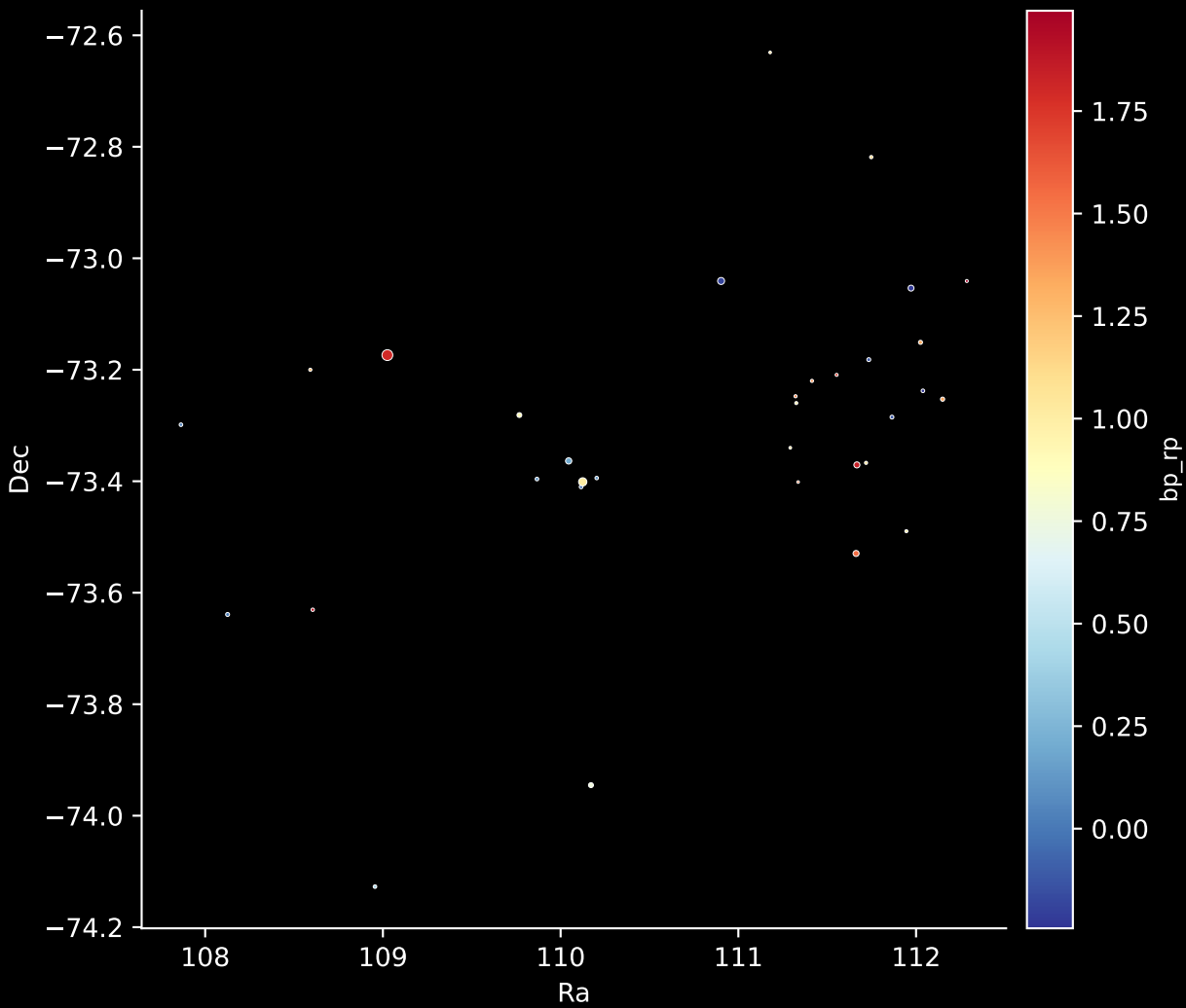
GALAH DR4 Field: [-7] Stars: 33
