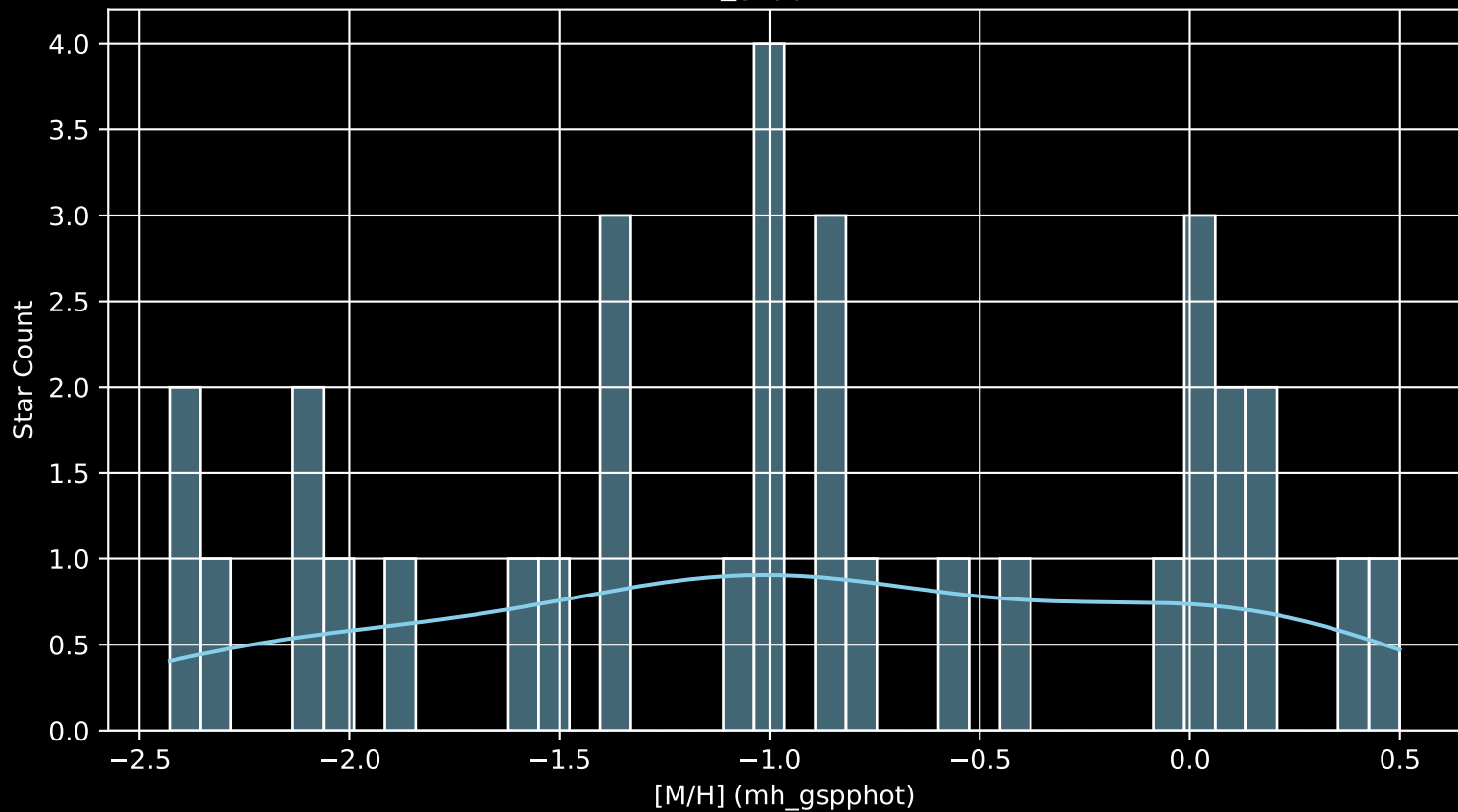
GALAH DR4 Field: [-7] [M/H] (mh_gspphot) (n= 33)
