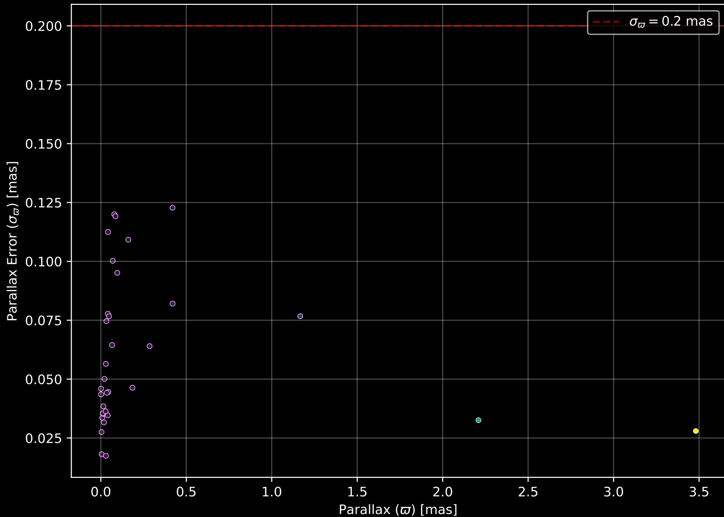
GALAH DR4 Field: [-7] Parallax Quality (n= 33)
